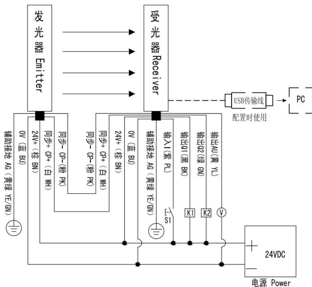
图 7-3 MCM 系列测量光栅 IQQAU 输出接线图
