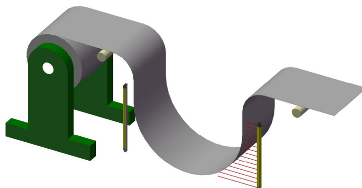
图 9-24 下垂度检测
