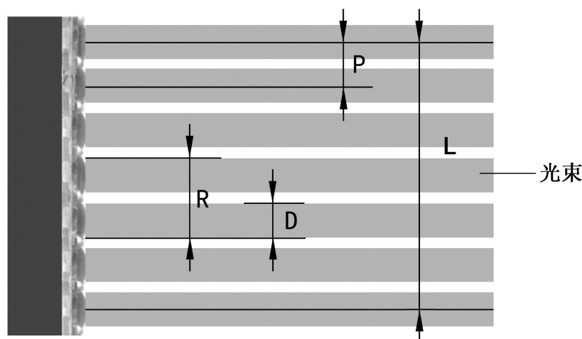
图 4-4 光轴间距与最小检出物体相关图解
