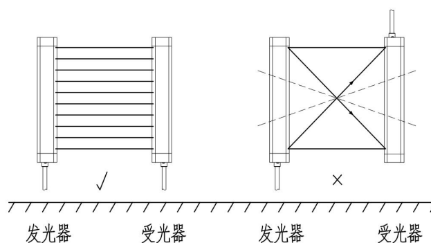
图 6-1 安装方向图示
