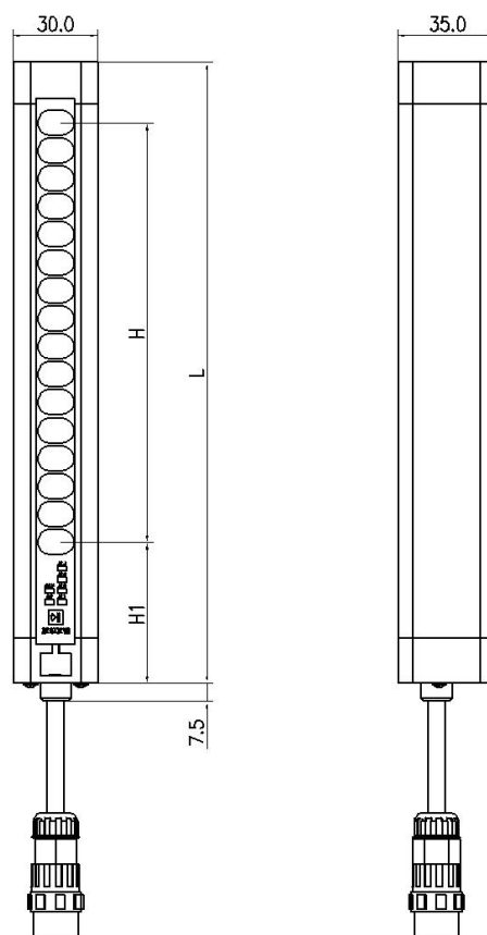
图 13-1 MCM 外形尺寸图
