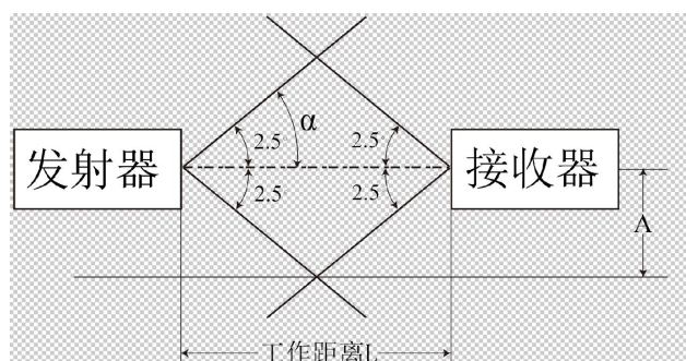
图 6-3 光束散射角
