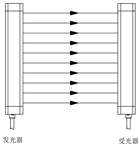
图 4-2 平行光束版本示意图
