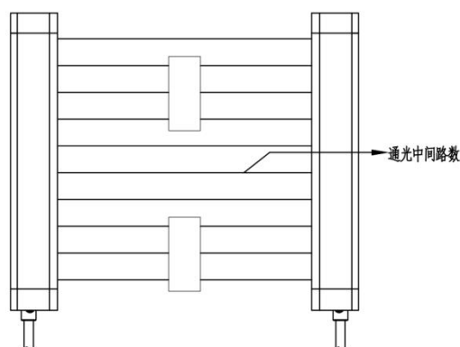
图 4-14 通光中间路数
