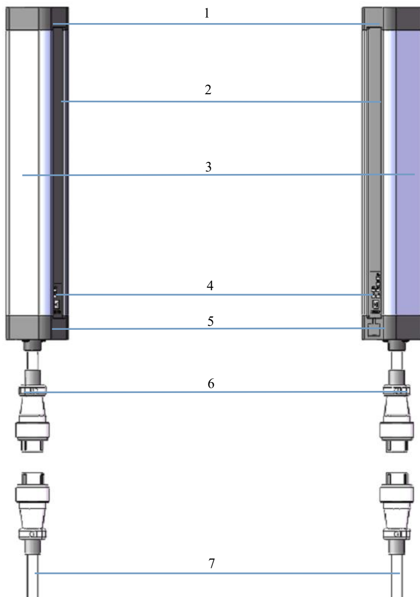
图 4-1 MCM 外观示意图
