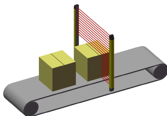
4-22 限高检测
