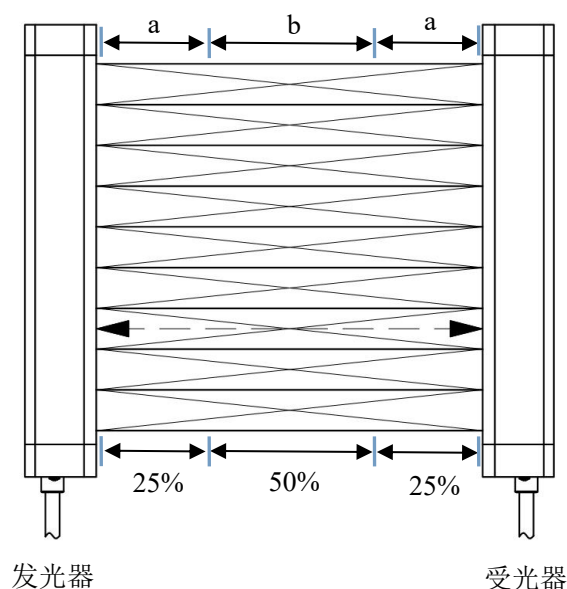
图 4-3 交叉光束版本示意图
