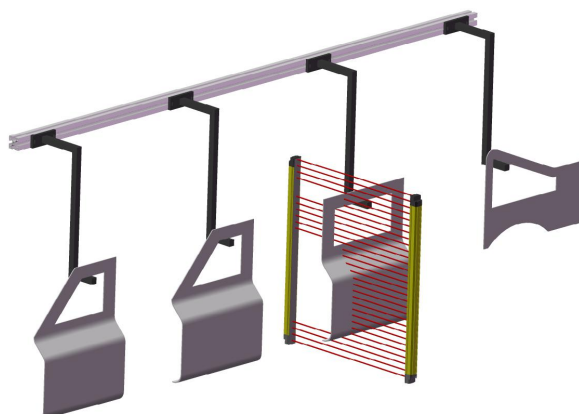
图 9-22 物体开窗大小检测
