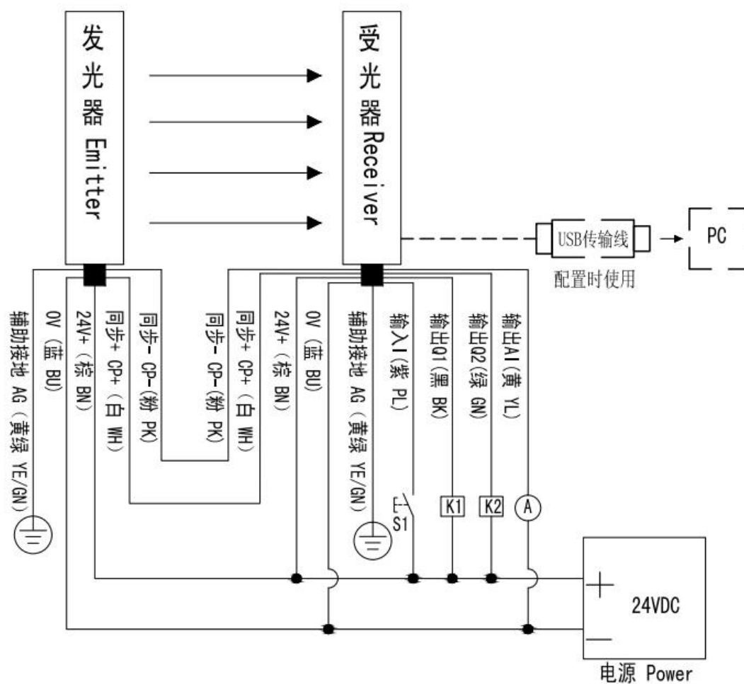
图 7-2 MCM 系列测量光栅 IQQAI 输出接线图
