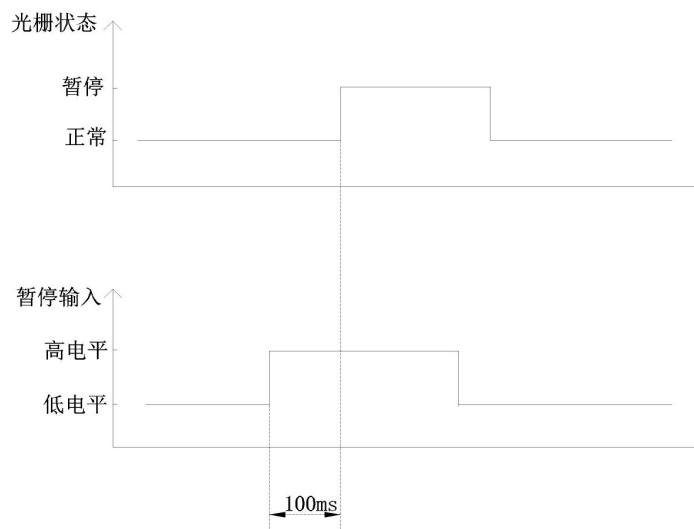
图 9-17 暂停功能输入与光栅状态示意图
