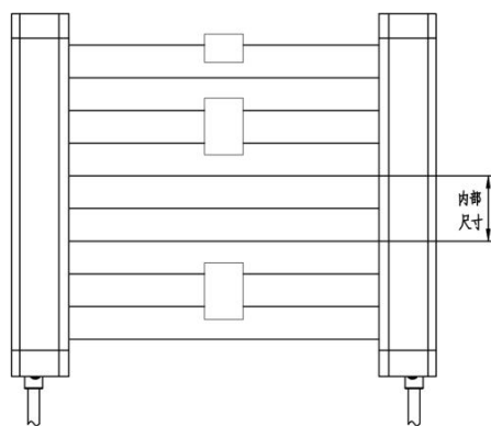
图 4-17 内部尺寸
