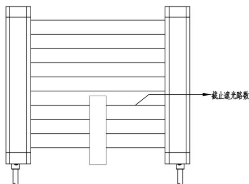
图 4-9 截止遮光路数
