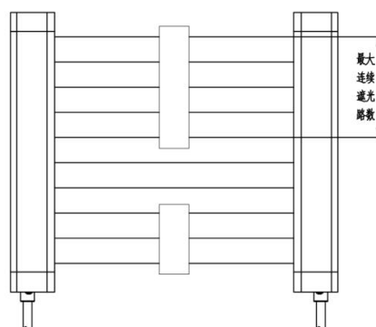
图 4-11 最大连续遮光路数
