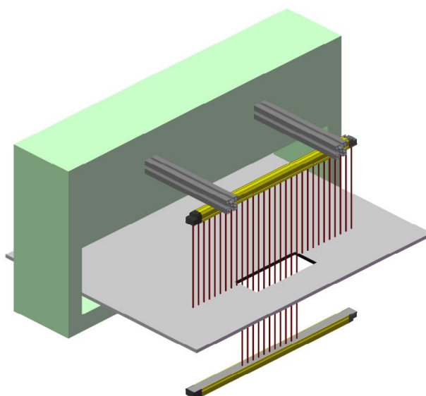
图 9-21 次品检出
