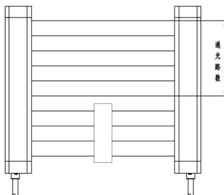
图 4-6 通光路数
