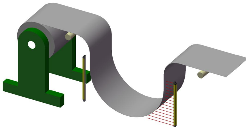
4-26 下垂度检测
