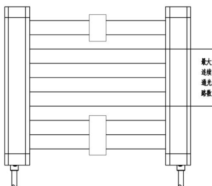
图 4-12 最大连续通光路数
