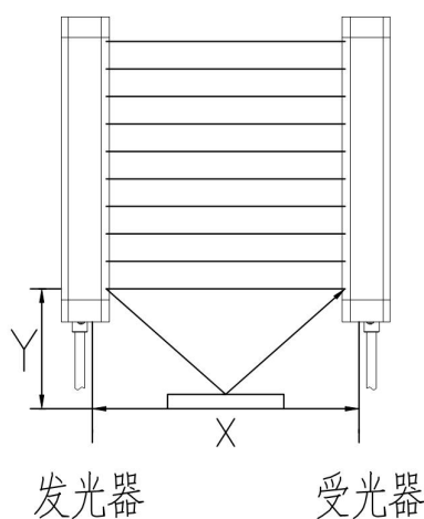
图 6-2 反射面对检测的影响
