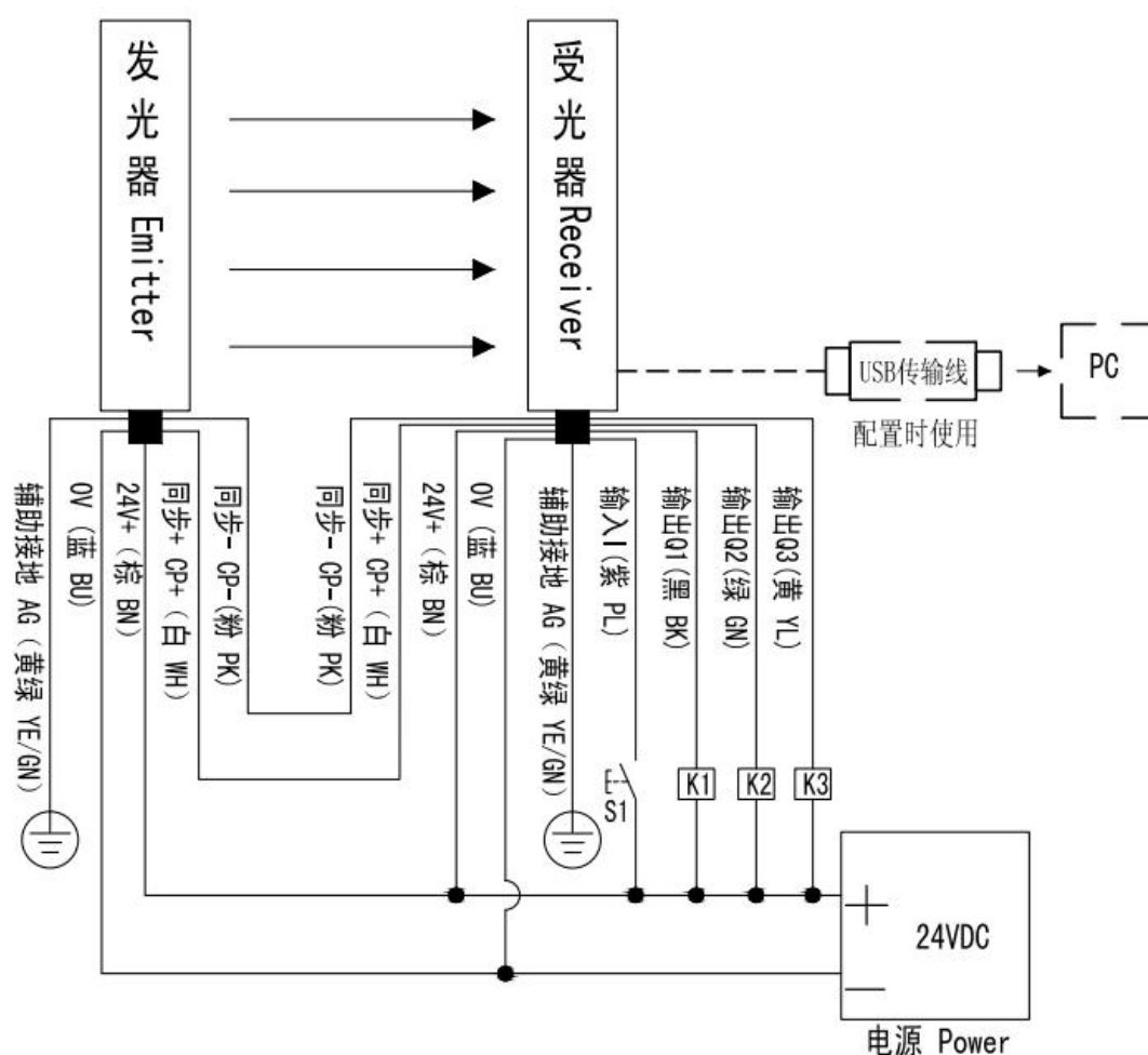
图 7-1 MCM 系列测量光栅 IQQQ 输出接线图
