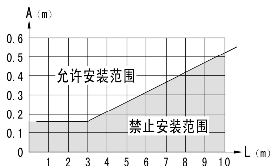
图 6-4 A 值确定坐标图
