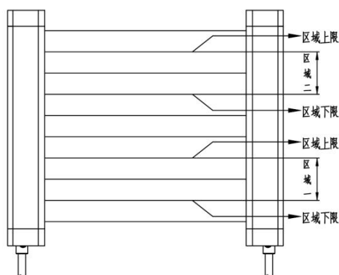
图 4-15 区域上下限
