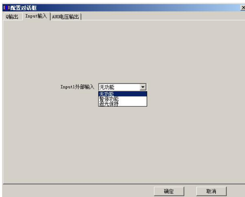
图 9-26 IQQAU 输入配置界面
