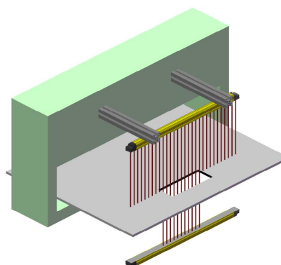
4-23 物料孔洞检测
