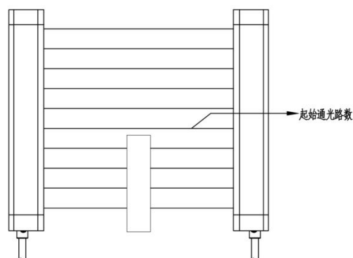
图 4-8 起始通光路数
